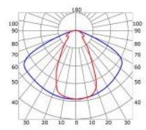
Lente 60° (riduzione luce: -16%)
