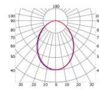
Diffusore nero (riduzione luce: -84%)
