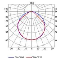
Diffusore trasparente (riduzione luce: -2%)
