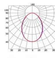
Diffusore nero (riduzione luce: -86%)
