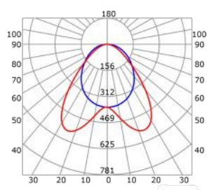
— C0-C180 — C90-C270 Lente con doppia asimmetria (riduzione luce -14%)
