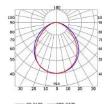
Diffusore semiopaco (riduzione luce: -9%)
