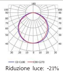
CURVA FOTOMETRICA
