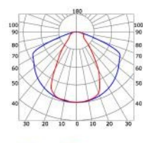
Lente 60° (riduzione luce: -3%)
