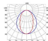
Diffusore semiopaco 67° (riduzione luce: -38%)
