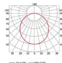
Diffusore opaco: -24% Diffusore satinato: -22%
