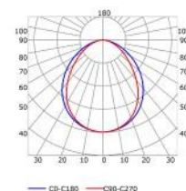
Diffusore semiotrasparente 90° (riduzione luce: -20%)
