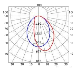
— C0-C180 — C90-C270 Lente asimmetrica (riduzione luce -21%)
