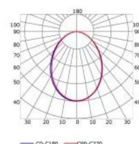
Diffusore nero (riduzione luce: -84%)
