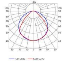
Diffusore trasparente 90° (riduzione luce: -16%)
