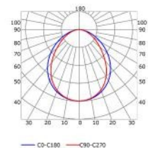
Diffusore semiopaco 90° (riduzione luce: -20%)
