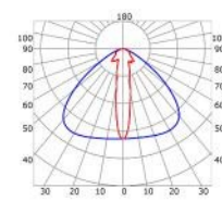
Lente 18° (riduzione luce: -34%)
