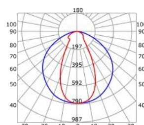
— C0-C180 — C90-C270 Lente 52° (riduzione luce -17%)
