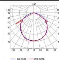
Diffusore trasparente (riduzione luce: -7%)
