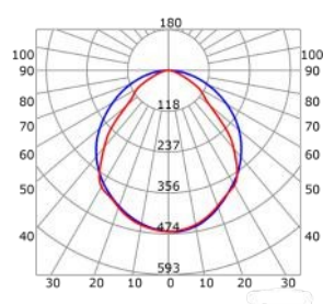
— C0-C180 — C90-C270 Lente 90° (riduzione luce -19%)
