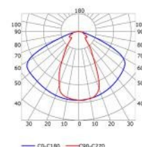
Lente 60° (riduzione luce: -16%)
