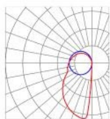
— C0-C180 — C90-C270 Diffusore satinato
