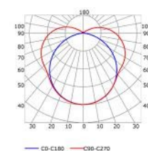
Diffusore opaco a L (riduzione luce: -25%)
